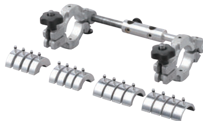
固定治具(二層管用) 20~50A
