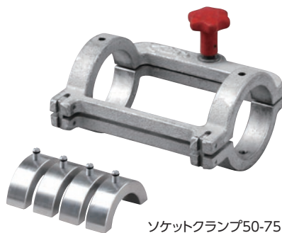
ソケットクランプ50-75
