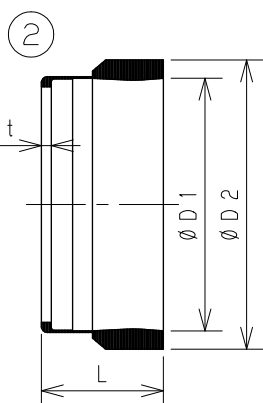
TM-II型パッキン寸法表
