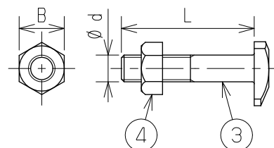
T字ボルト・ナット寸法表
