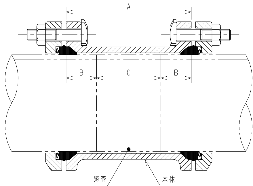
組立図
