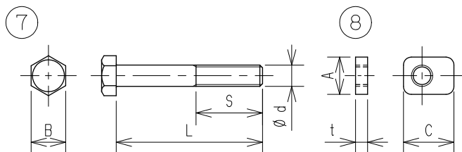
SUS製六角ボルト・LKナット寸法表 単位：mm
